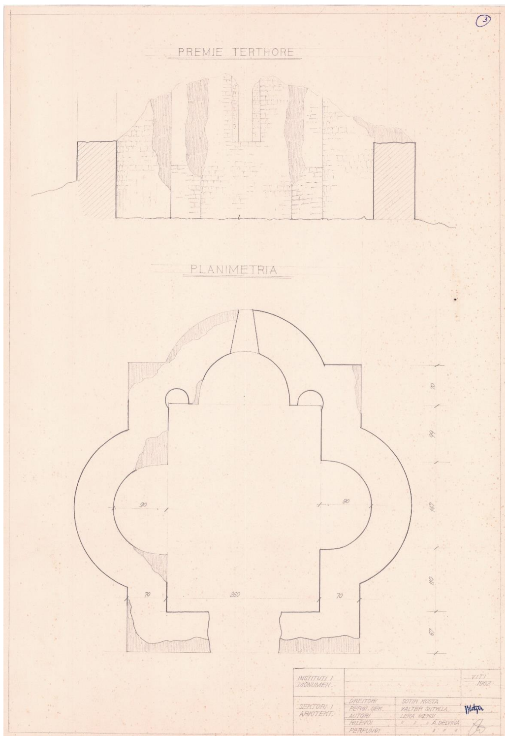
Foto 4. Prerje dhe planimetria e kishës. Burimi: Arkiva IKTK
